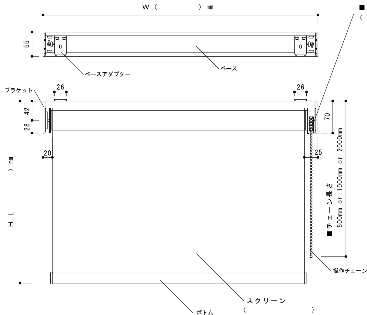
【ベースアダプター寸法】
