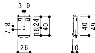
【ベースアダプター寸法】
