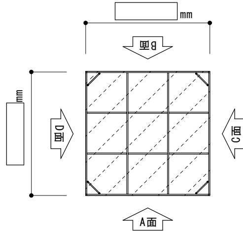
屋根伏図
