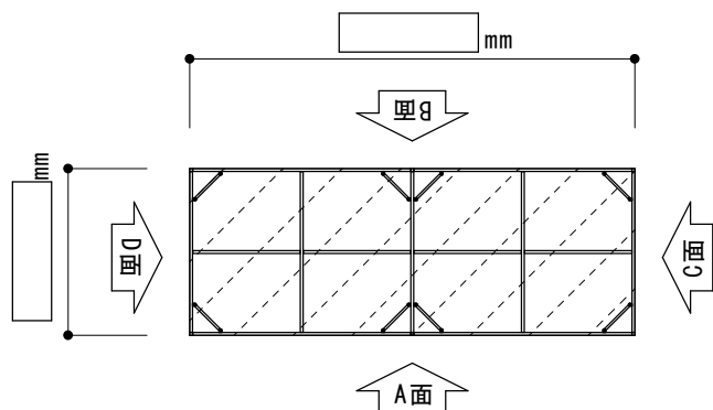
屋根伏図
