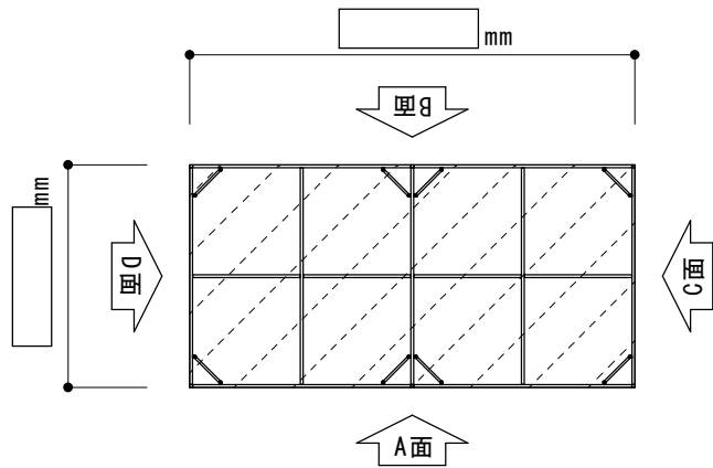
屋根伏図
