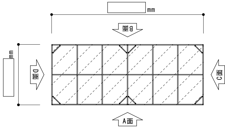
屋根伏図
