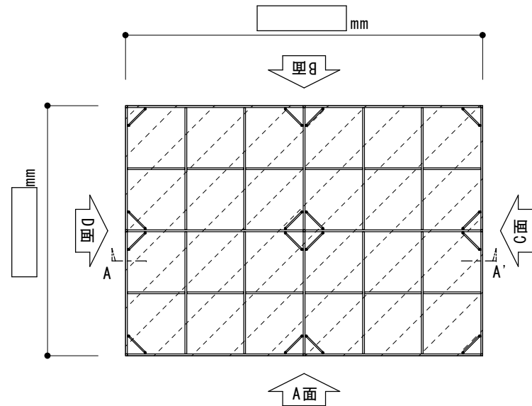
屋根伏図
