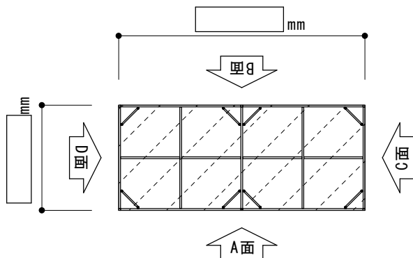
屋根伏図
