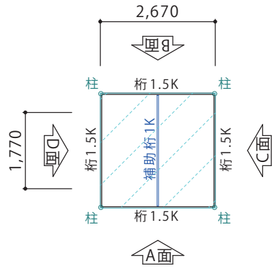
屋根伏図
