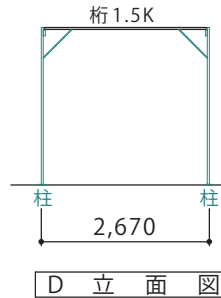
D 立面図
