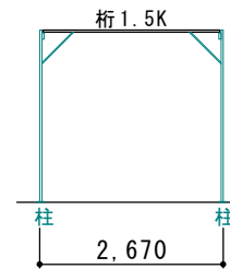
D立面図
