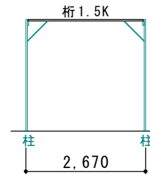
C立面図
