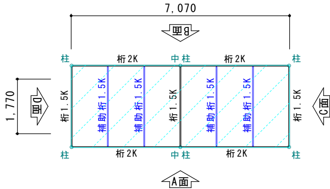
屋根伏図
