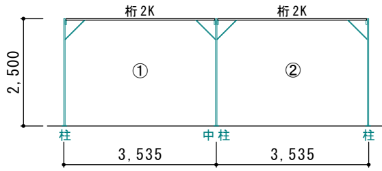
A立面図
