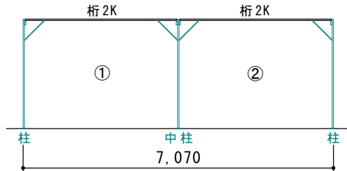
B立面図
