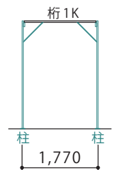
C 立面図
