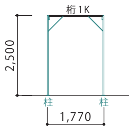
A 立面図
