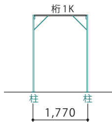
B 立面図
