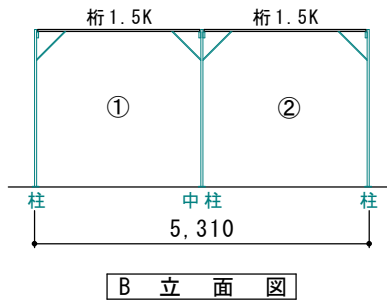
B 立面図
