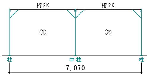
B 立面図
