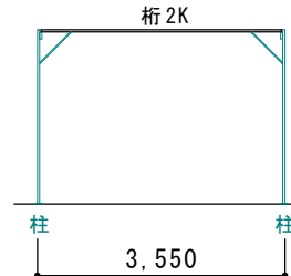
C 立面図
