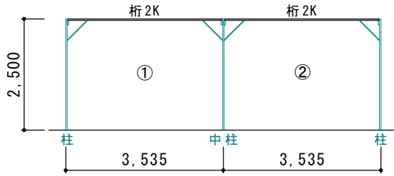
A 立面図
