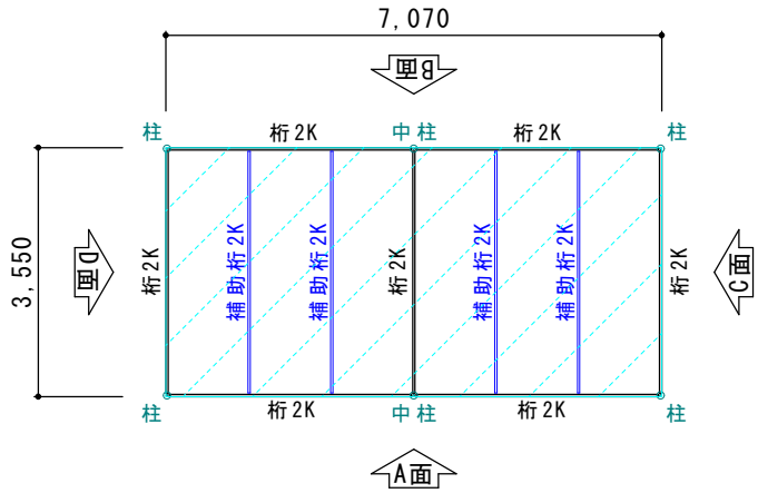
屋根伏図
